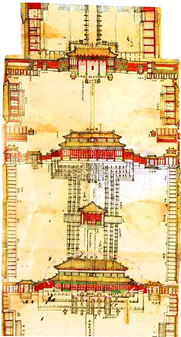
大清门至坤宁宫中一路图样（局部） 清 “样式雷”家族
