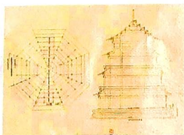
颐和园佛香阁平面地盘样、大木立样 清 “样式雷”家族
